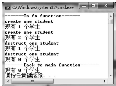
图 3.28 例 3.19 的运行结果
