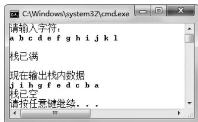
图 3.5 例 3.3 的运行结果
