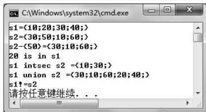
图 3.33 例 3.22 的运行结果
