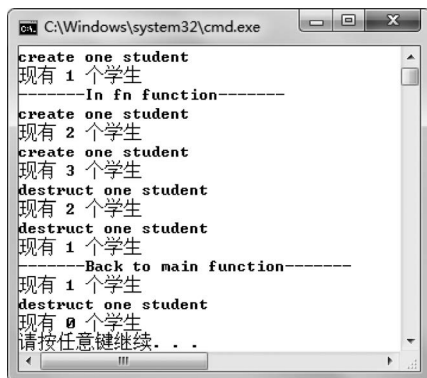
图 3.29 修改例 3.19 后的运行结果
