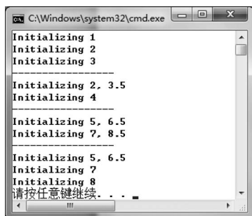
图 3.16 例 3.11 的运行结果
