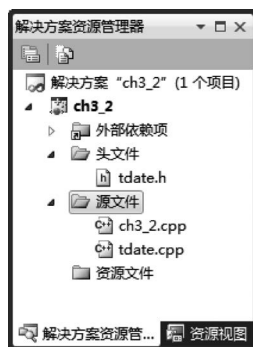
图 3.1 例 3.1 项目文件结构
