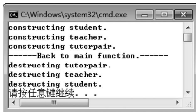
图 3.26 例 3.17 的运行结果
