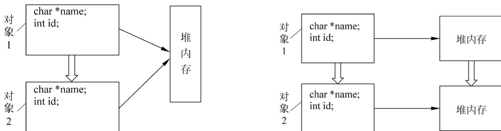
图 3.17 浅拷贝的两种情况示意图
