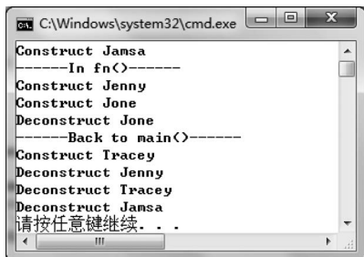
图 3.30 例 3.20 的运行结果
