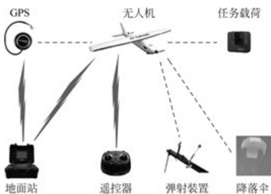
图 1-1 一种典型的无人机系统
