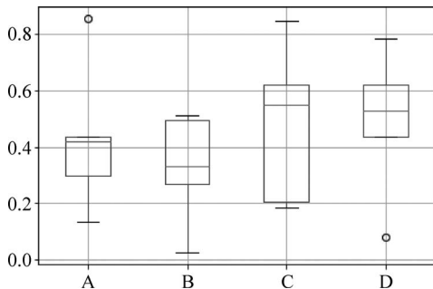
图 3-3 绘制箱线图
