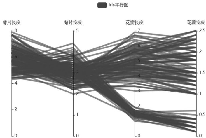
图 3-6 平行坐标图
