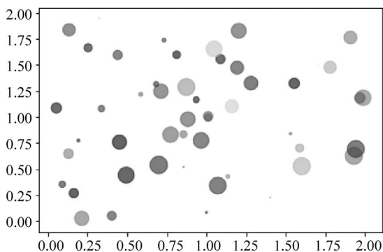
图 3-4 三维散点图
