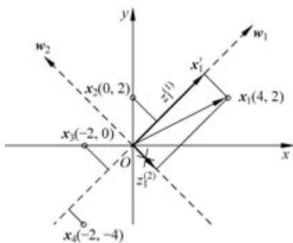
图 5-4 二维平面上的主成分分析示例
