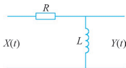
图 3.32 RL 电路
