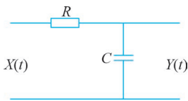
图 3.29 RC 电路
