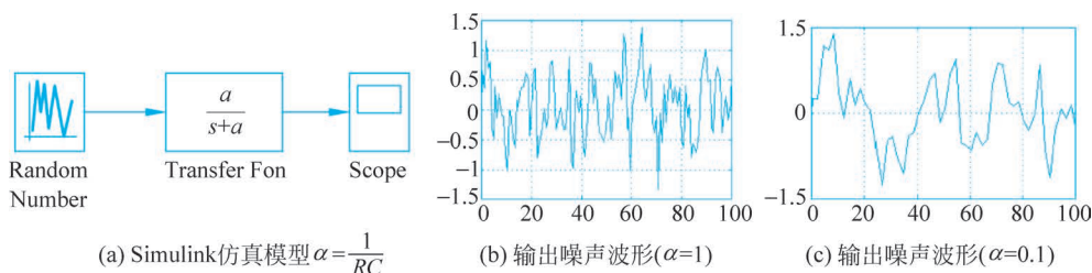
图 3.14 白噪声通过 RC 电路的 Simulink 仿真模块
