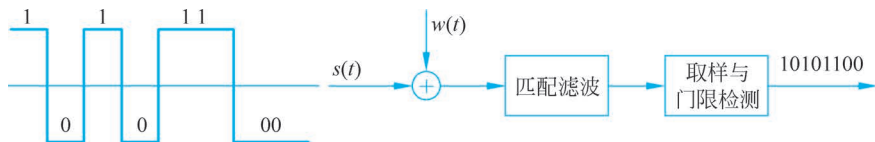
图 3.37 匹配滤波器在二元 PAM 信号传输中的应用
