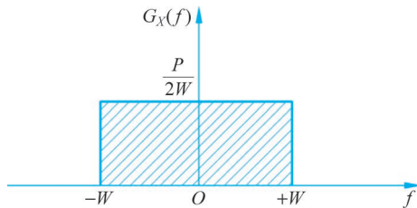
图 3.35 功率谱密度
