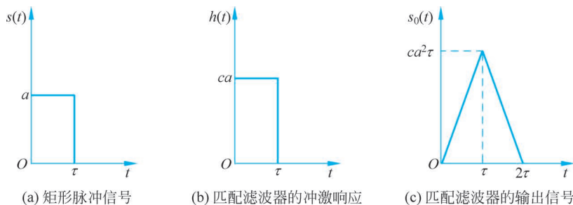
图 3.20 矩形脉冲的匹配滤波器
