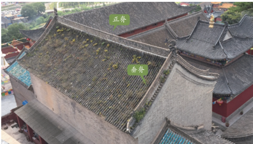
硬山顶各部分示意图（五台山）
